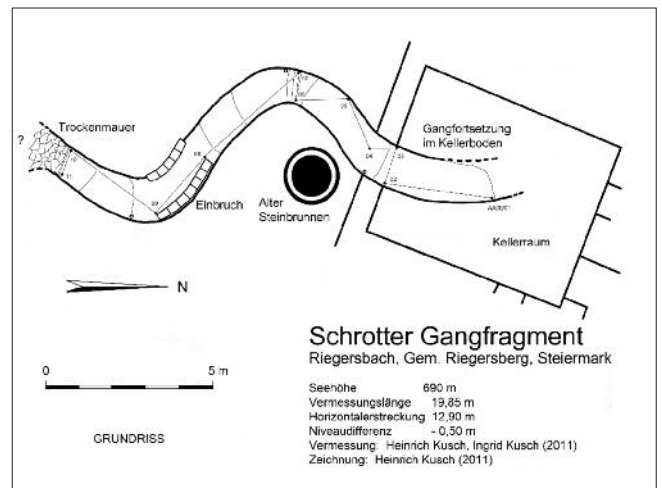
Abb. 5: Grundrissplan des Schrotterganges bei Riegersbach • Floor plan of Schrottergang at Riegersbach. Zeichnung: Dr. Heinrich Kusch
