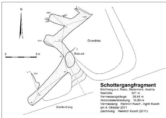
Abb. 15: Grundrissplan des Schottergangfragmentes • Floor plan of Schottergangfragment ; Zeichnung: Heinrich Kusch
